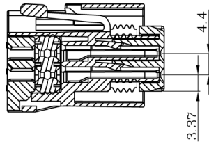
SECTION D-D
